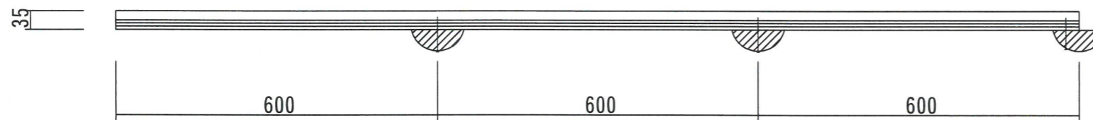
平面図 S=1:10 . . .
