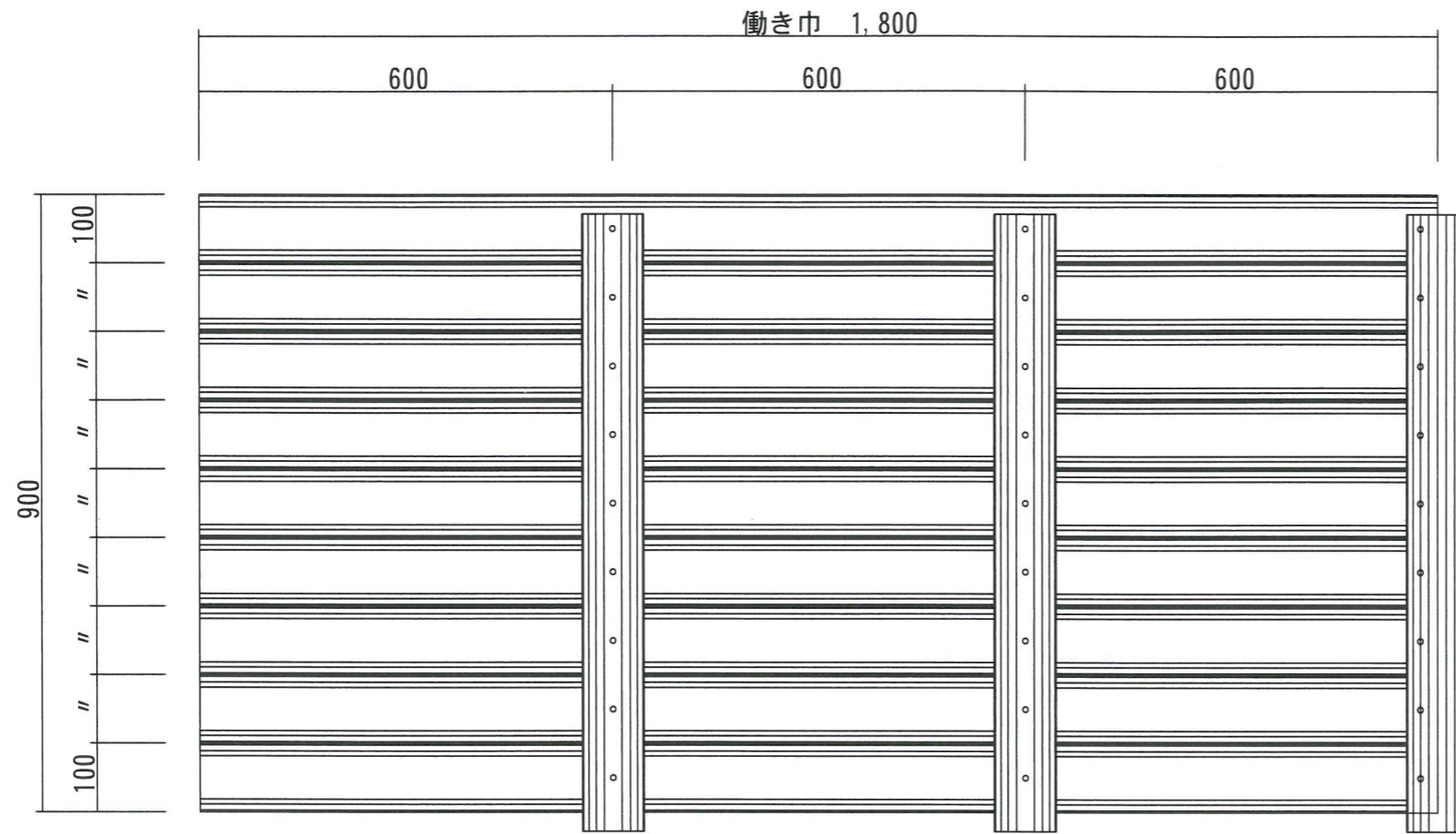
正面図 S=1:10 . . .
