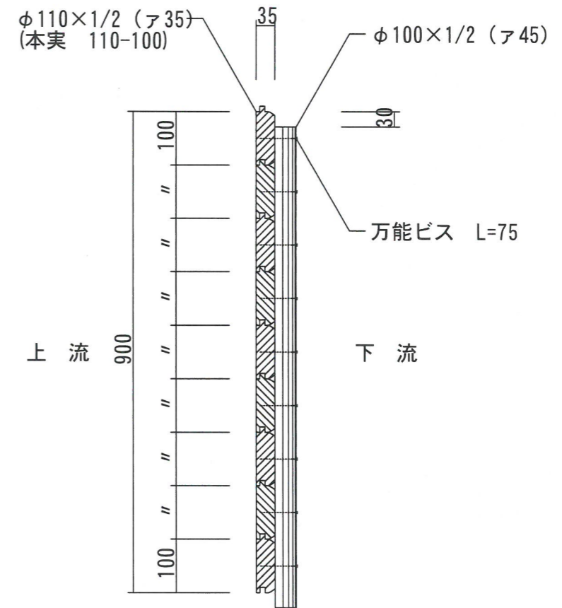
断面図 S=1:10 . . .
